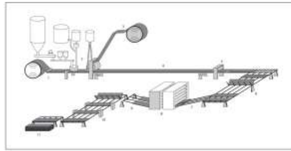
Abbildung 1: Fertigungsprozess von Gipsplatten nach /Gips-Datenbuch/
